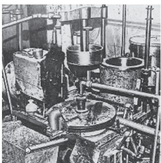
上: 1931年(昭和6)当時のクレパス 下: クレパス製造機械の第1号機
